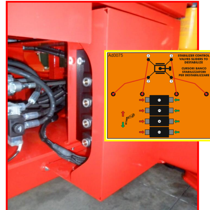
Figure 36 : poste stabilisateurs.
